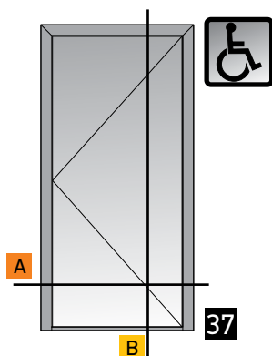
Single leaf door inward opening with windbreak Μονόφυλλη πόρτα ανοιγόμενη μέσα με ανεμοφράχτη
