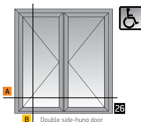
Double side-hung door inward opening without threshold Δίφυλλη πόρτα ανοιγόμενη μέσα με λάστιχο χωρίς κατωκάσι
