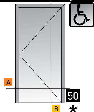
Single leaf door inward opening, hidden sash with threshold Μονόφυλλη πόρτα ανοιγόμενη μέσα, κρυφό φύλλο με χαμηλό κατωκάσι
