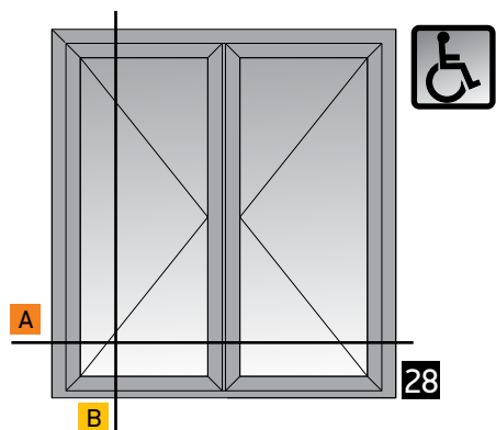
Double side-hung door inward opening with windbreak Δίφυλλη πόρτα ανοιγόμενη μέσα με ανεμοφράχτη
